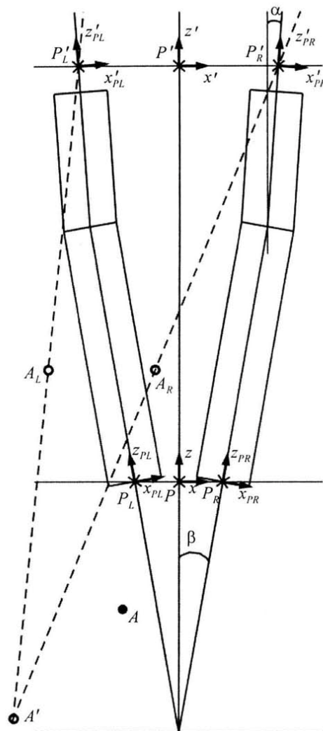
Рис. 1. Схема формирования стереоскопического изображения в стереомикроскопе Грену. PP' – ось симметрии стереомикроскопа; x, y, z и x', y', z' – системы координат пространства предметов и пространства изображений. Остальные пояснения см. в тексте.
